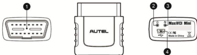
Рисунок 2-4 Беспроводной диагностический интерфейс MaxiVCI Mini
